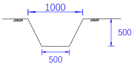
土质沉沙池断面图
