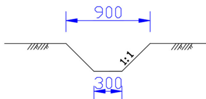
土质排水沟A-A断面图
