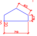
侧面上六边形骨架盖板侧视图
