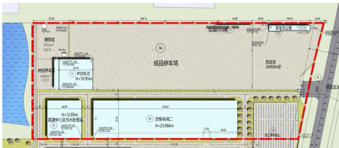
图 2.1 厂区总平面布置图
