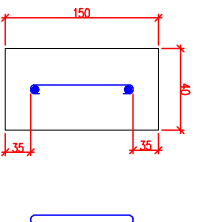
A-A剖面图
