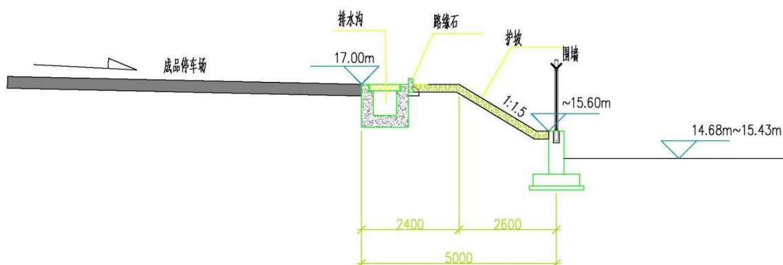
图 3.1 成品停车场至围墙处护坡断面
