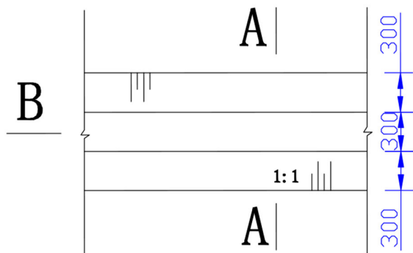
土质排水沟平面图
